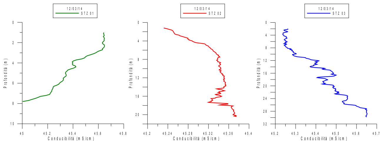
Fig. 5 Andamento della Conducibilità nelle Stazioni ST01PT, ST02PT, ST03PT durante la campagna FPOA_5
