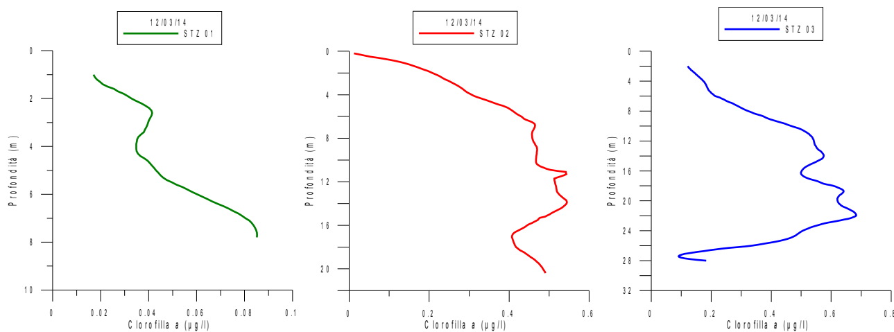
Fig. 9 Andamento della Clorofilla a nelle Stazioni ST01PT, ST02PT, ST03PT durante la campagna FPOA_5
