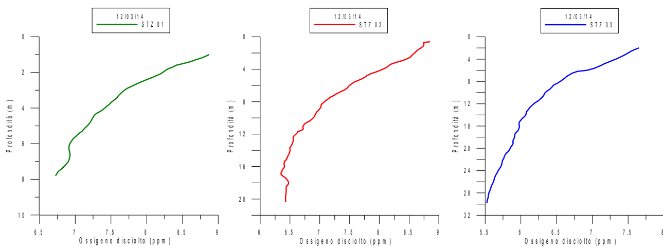
Fig. 8 Andamento dell'Ossigeno disciolto nelle Stazioni ST01PT, ST02PT, ST03PT durante la campagna FPOA_5
