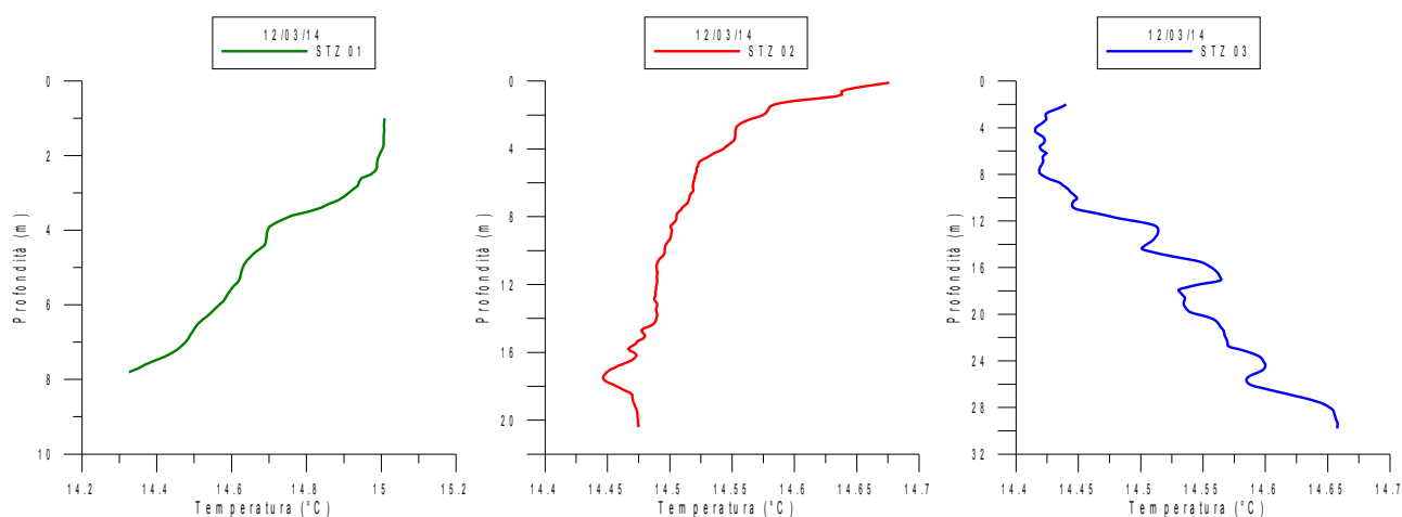
Fig. 4 Andamento della Temperatura nelle Stazioni ST01PT, ST02PT, ST03PT durante la campagna FPOA_5
