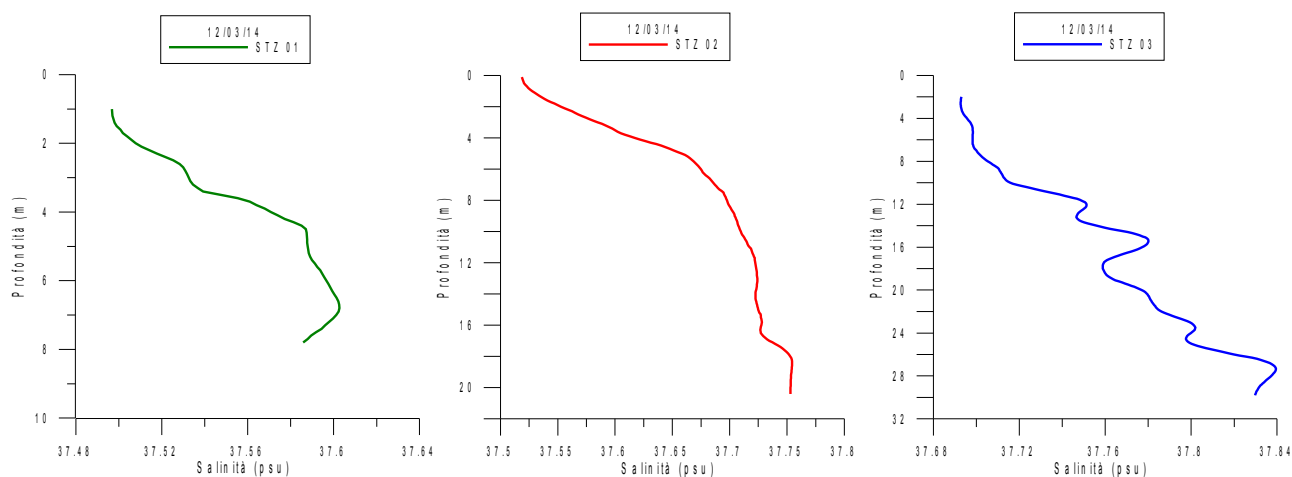
Fig. 6 Andamento della Salinità nelle Stazioni ST01PT, ST02PT, ST03PT durante la campagna FPOA_5
